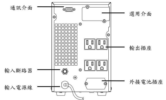
↑ 圖1-1 C-1000F(S)後蓋板
