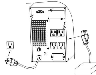
↑ 圖2-2 C-1000F(S)~C-3000F(S)、C-1000RN輸出插座接線方式示意圖
