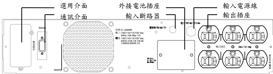
↑圖 1-4 C-1000RN 後蓋板
