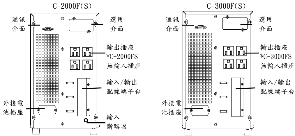
↑圖 1-2 C-2000F(S)、C-3000F(S)後蓋板
