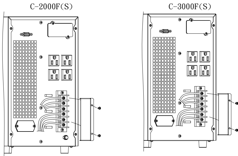
↑圖 2-3 C-2000F(S)/C-3000F(S)輸入、輸出端子排連接方式示意圖
