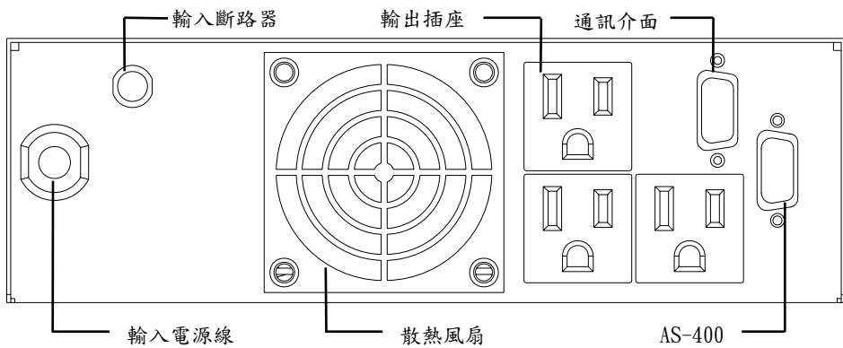
↑圖 1-5 C-1000RN 後蓋板(未內含電池型)
